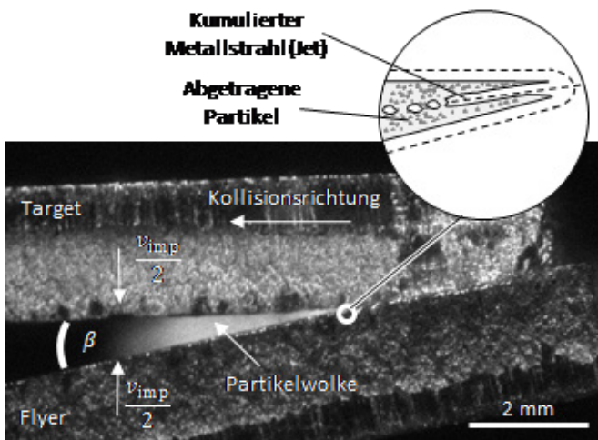
[2] Hochgeschwindigkeitsaufnahme des Fügespalts während des Kollisionsschweißprozesses; im Detail: Ausbildung des Jets als kumulierter Strahl und der Partikelwolke durch abgetragene Partikel
