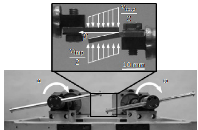
[1] Funktionsweise des Modellversuchsstands: zwei angetriebene Rotoren bringen zwei an die Enden montierte Fügepartner unter einer Aufprallgeschwindigkeit v_{imp} und einem Kollisionswinkel \beta definiert zur Kollision.
