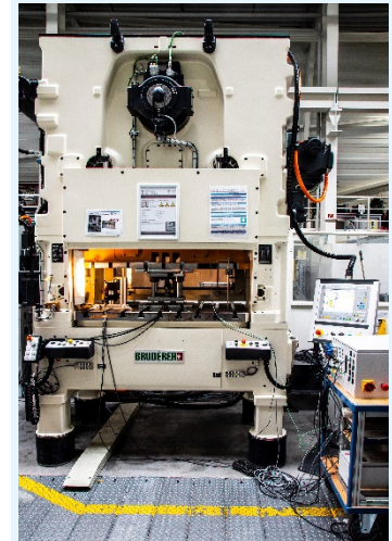
Betreuung der industriellen Versuchsanlage Bruderer BSTA 810
